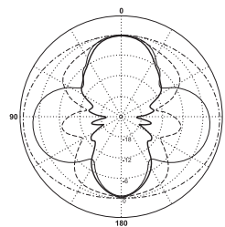
Piano orizzontale
